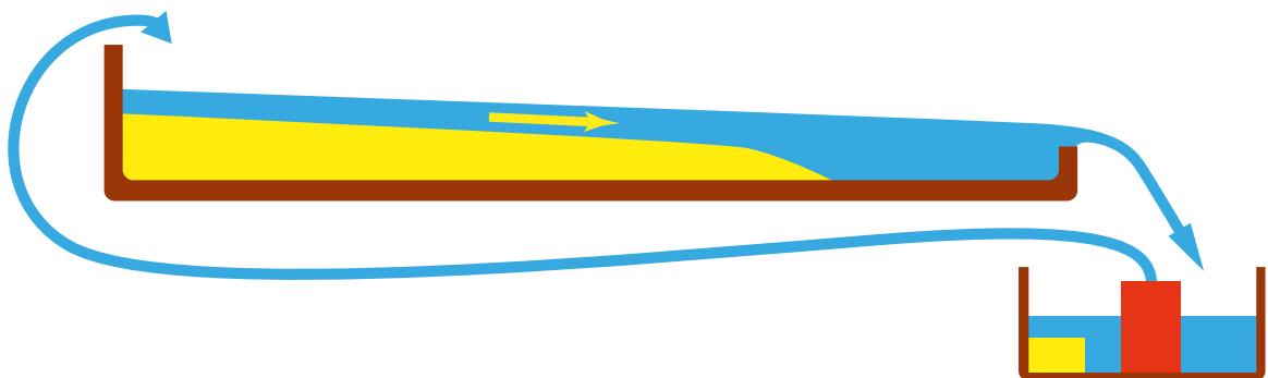
Fig.2a: Schematisch zijaanzicht van de stroomgootopstelling: bak (bruin) met zand (geel), water (blauw), waterkringloop (blauwe pijlen) via de pomp (rood) en de opvangbak (bruin, rechthoekig)
