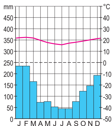
klimaatgrafiek d
