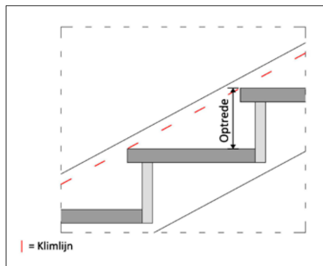
Figuur 2.6: Klimlijn
