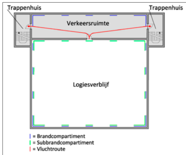
Figuur 3.17: Verkeersruimte beschermde vluchtroute
