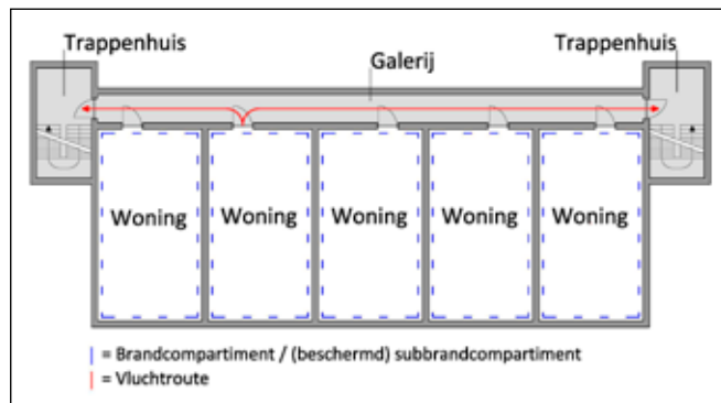
Figuur 3.1: Woongebouw met galerij
