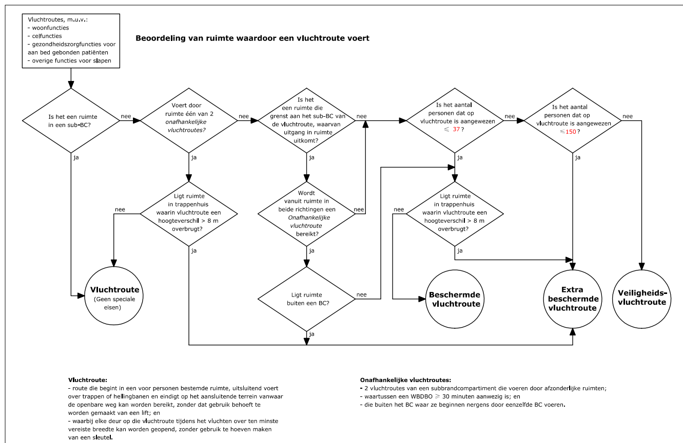
Stroomschema kantoorgebouw algemeen
