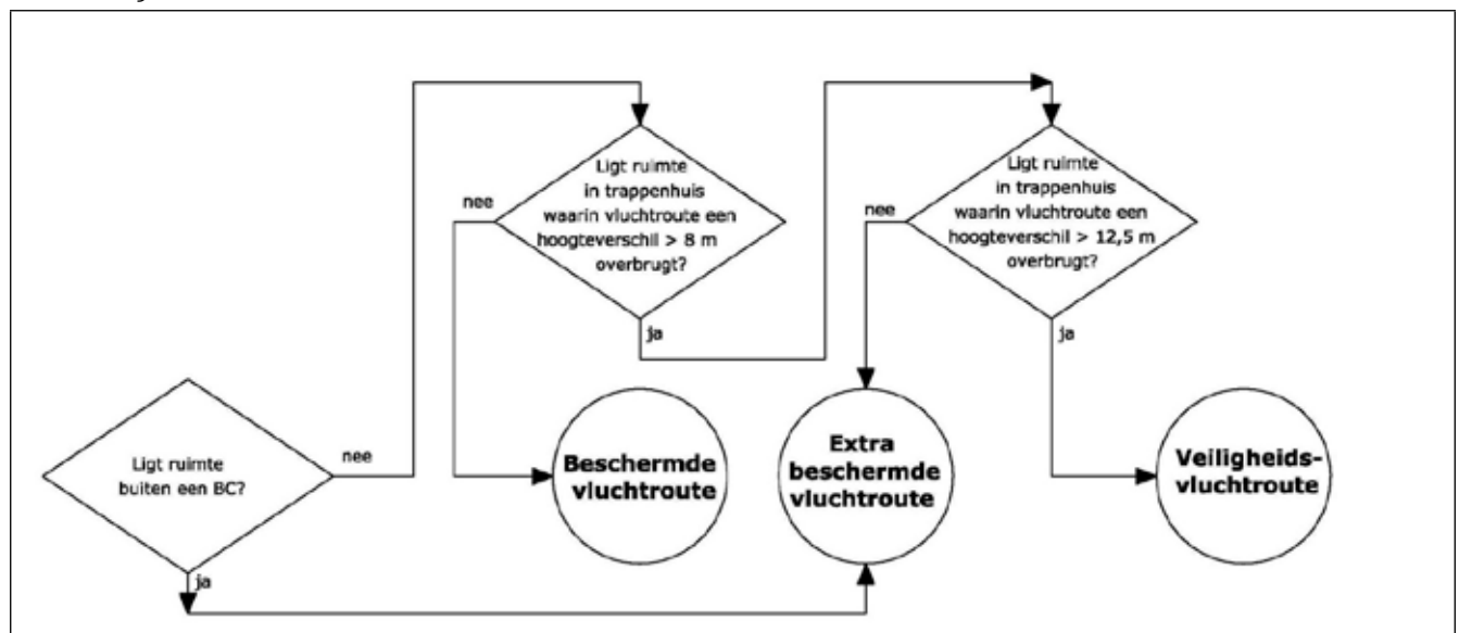
Stroomschema 3d.D
