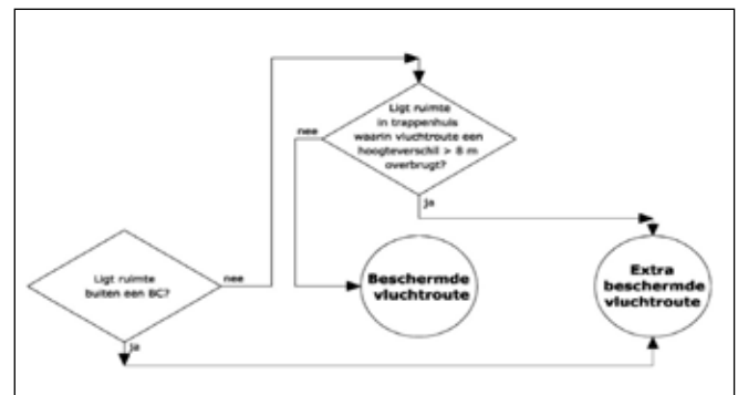
Stroomschema 3c.D
