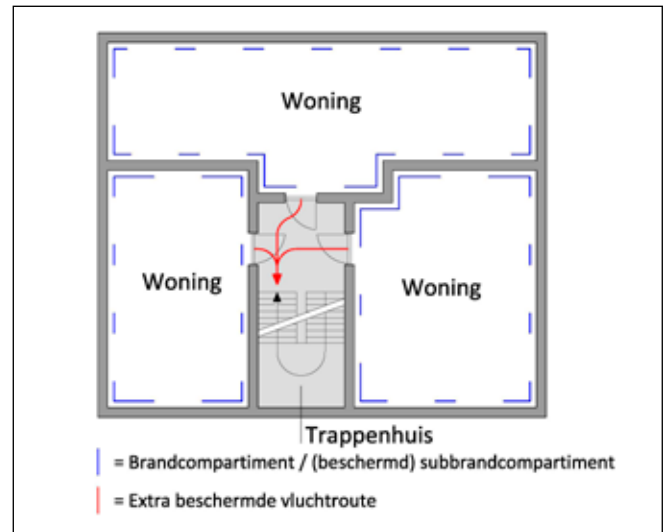
Figuur 3.6: Portieketageontsluiting
