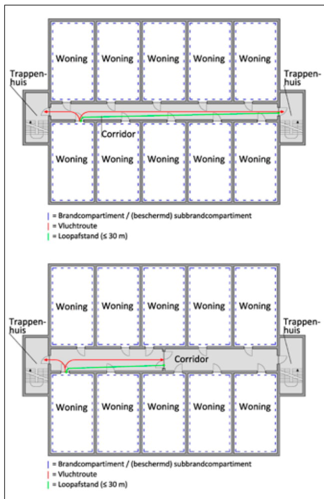
Figuur 3.2a en 3.2b: Woongebouw met corridor
