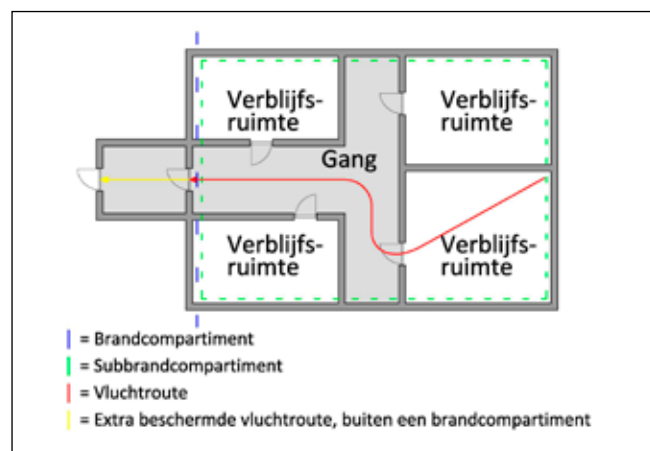
Figuur 2.3: Extra beschermd vluchtroute
