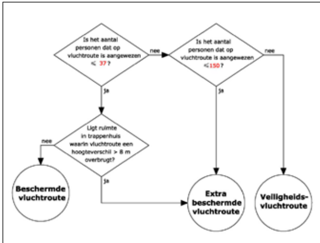
Stroomschema 3c.E
