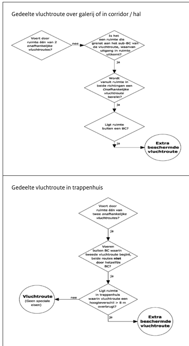
Stroomschema 3a.B
