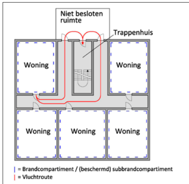
Figuur 2.4: Veiligheidsvluchtroute
