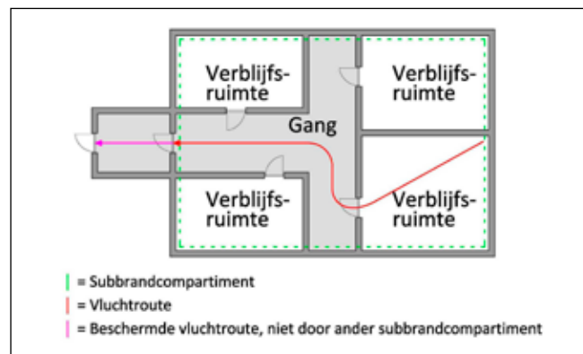
Figuur 2.2: Beschermd vluchtroute
