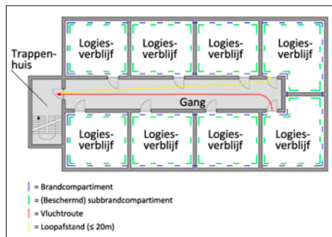
Figuur 3.18: Logiesfunctie met doodlopend eind
