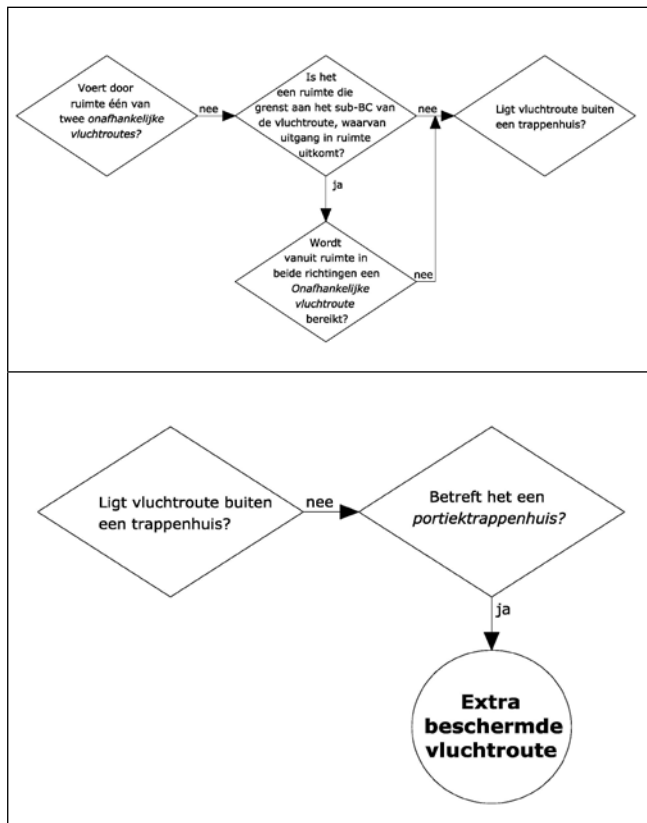
Stroomschema 3a.E
