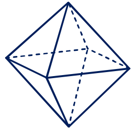
achtvlak octaeder
