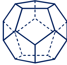
twaaflvlak dodecaeder
