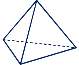
viervlak tetraeder
