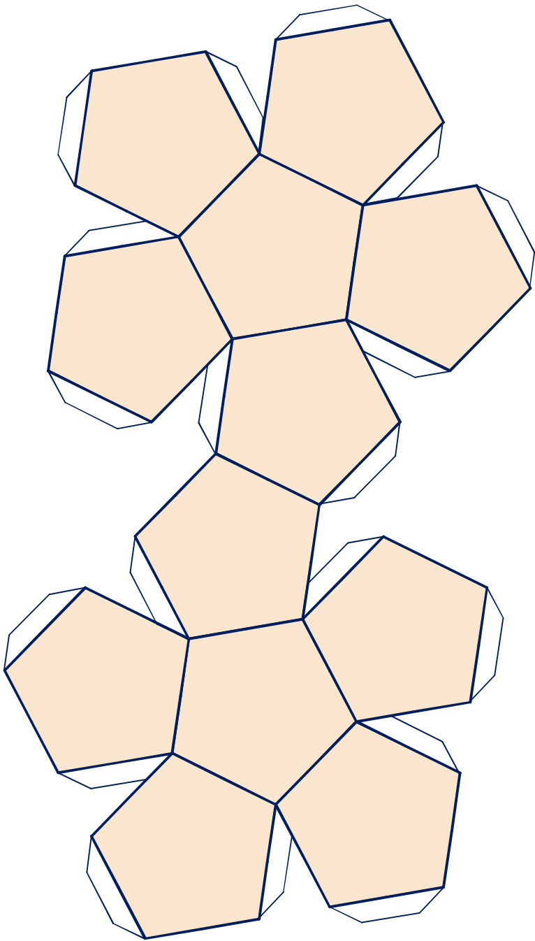
twaaflvlak dodecaeder
