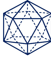
twintigvlak icosaeder
