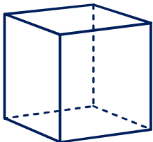
zesvlak hexaeder
