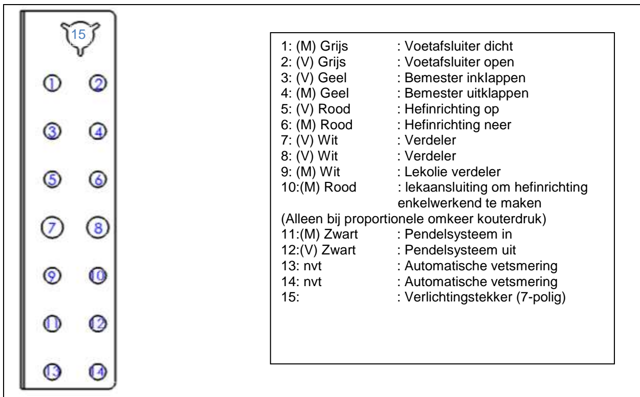
Figuur 4-1 schematische weergave hydr slangen bemester
