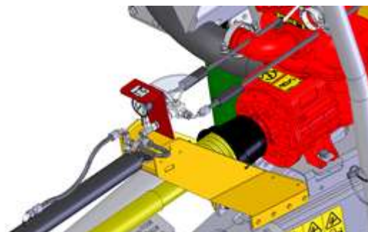
Figuur 5-1 Drukloos zetten topdrukcilinder
