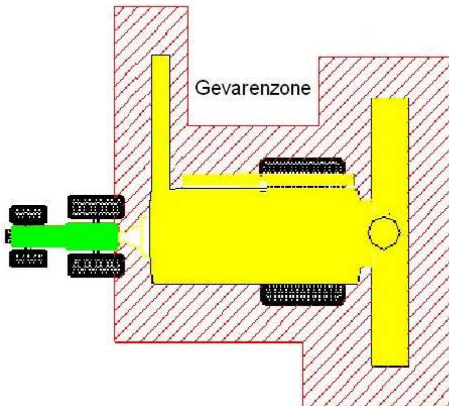
Figuur 3-1 gevarenzone rondom machine
