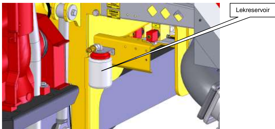
Figuur 5-3 lekreservoir hydr systeem
