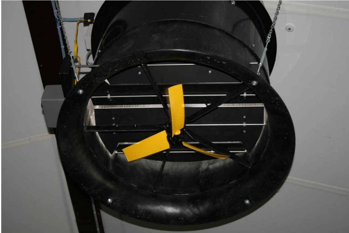
Figuur 11 Ventilator met meetwaaier en smookklep
