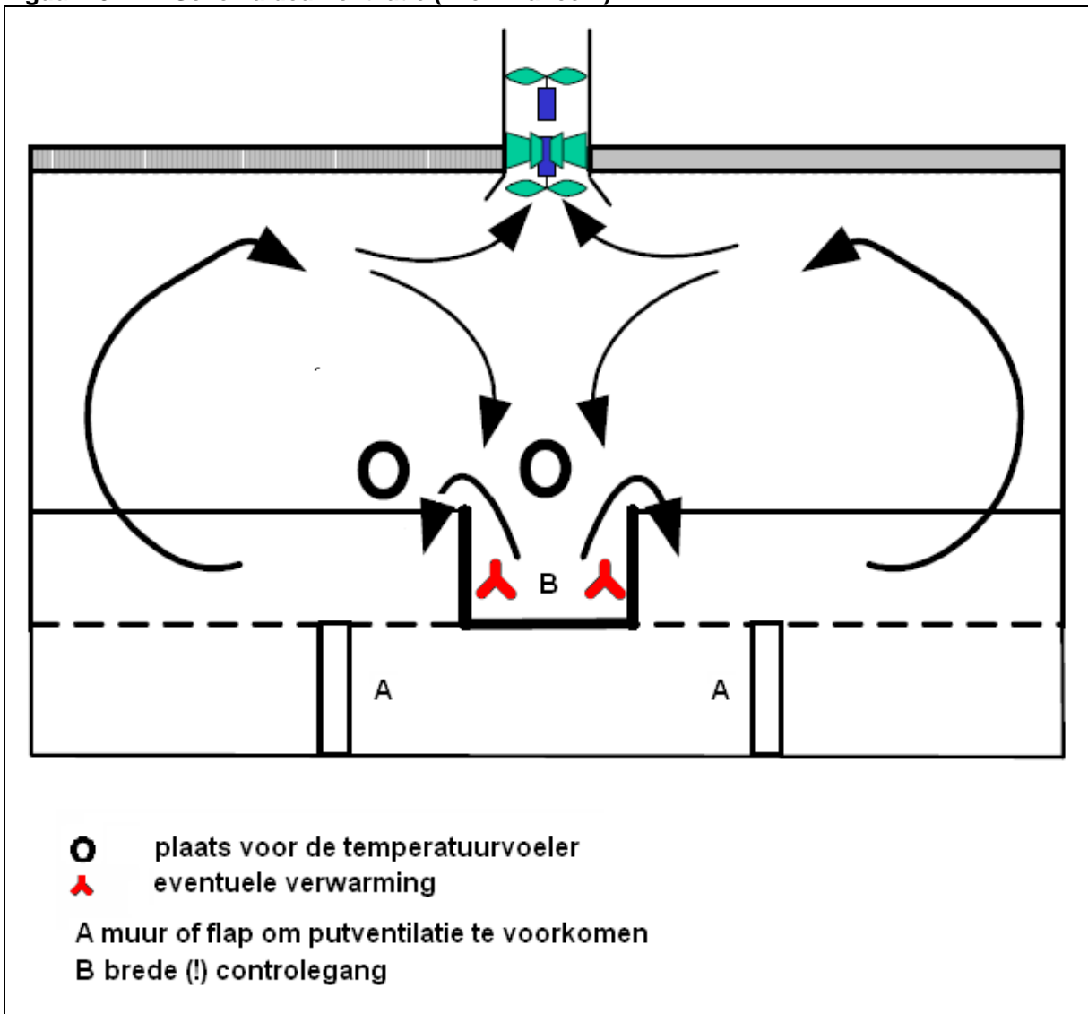
Figuur 20 Doorsnede deurventilatie (bron: Klimaatplatform varkenshouderij)
