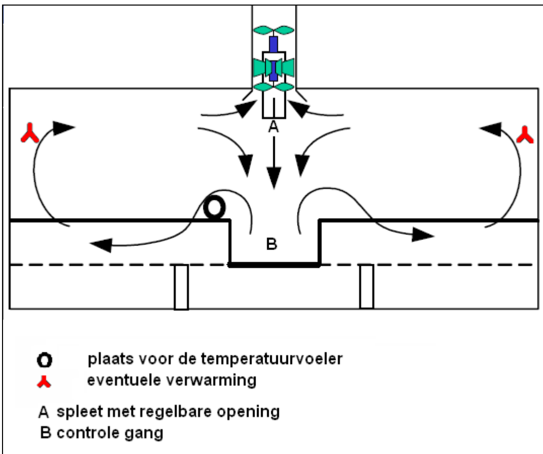
Figuur 30 Doorsnede combiventilatie (Bron: Klimaatplatform varkenshouderij)
