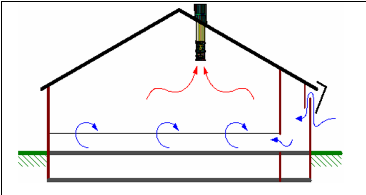
Figuur 19 Schema deurventilatie (Bron: Fancom)
