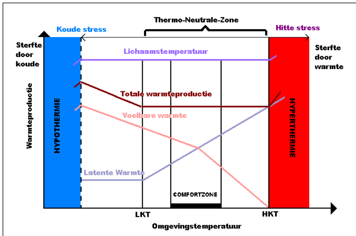
Figuur 3 Thermoregulatie van varkens en temperatuurzones
