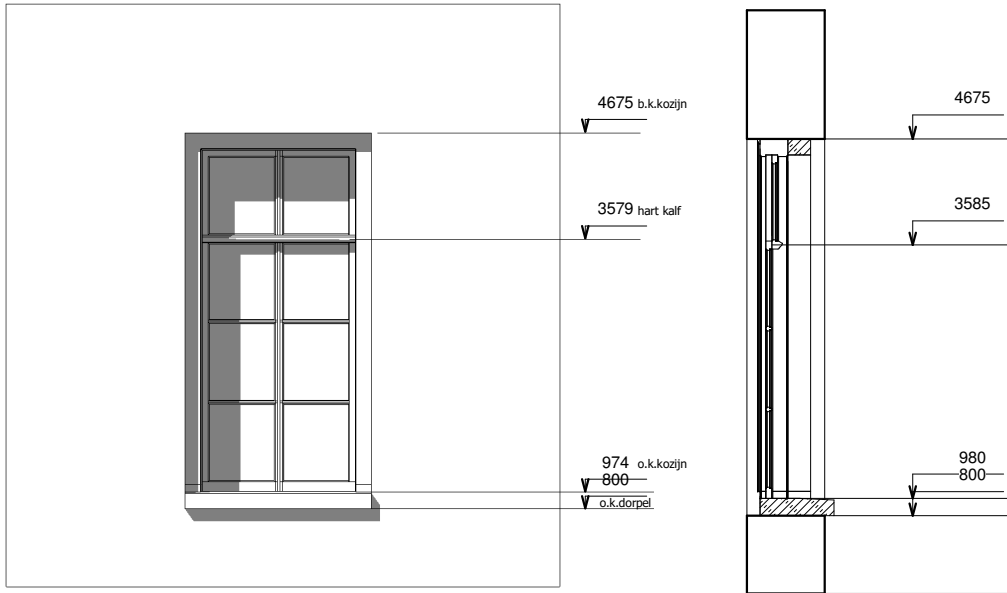
Aanzicht voor
