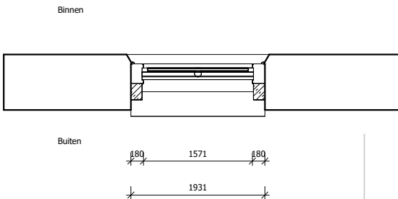
Aanzicht boven
