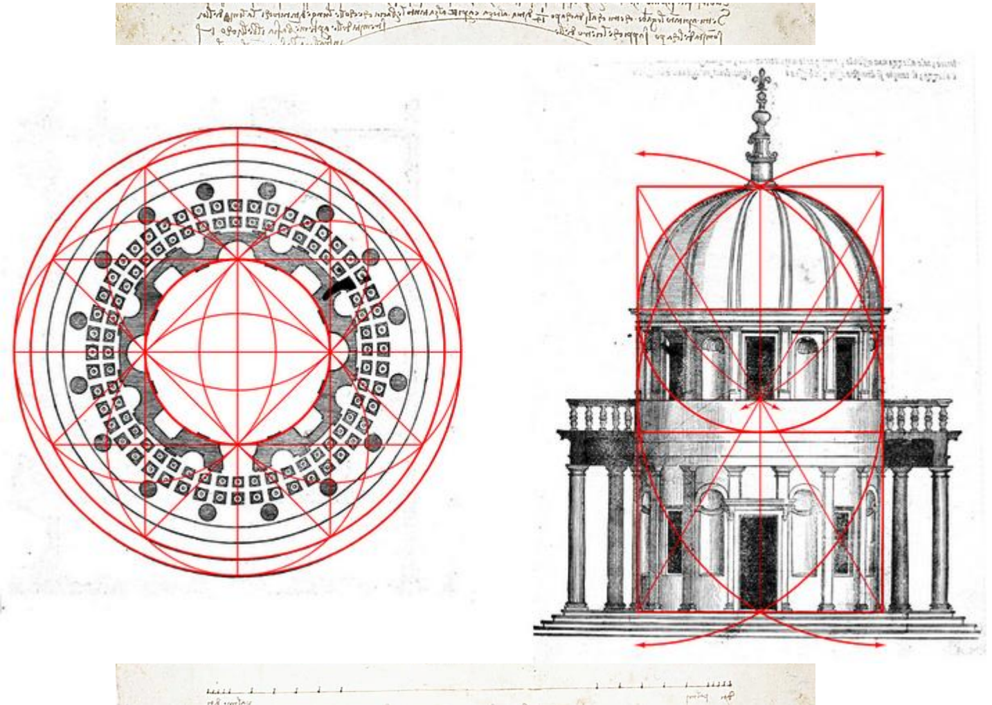
Tempietto, Bramante 1502
