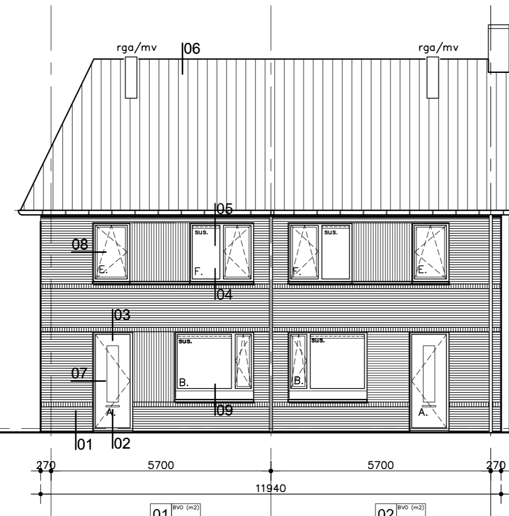
Zuidwestgevel kavel 01 en 02
