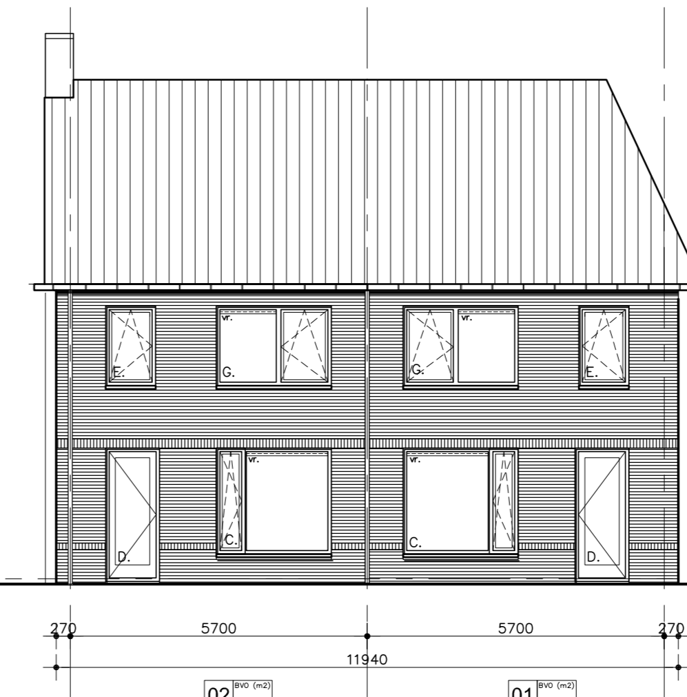
Noordoostgevel kavel 01 en 02
