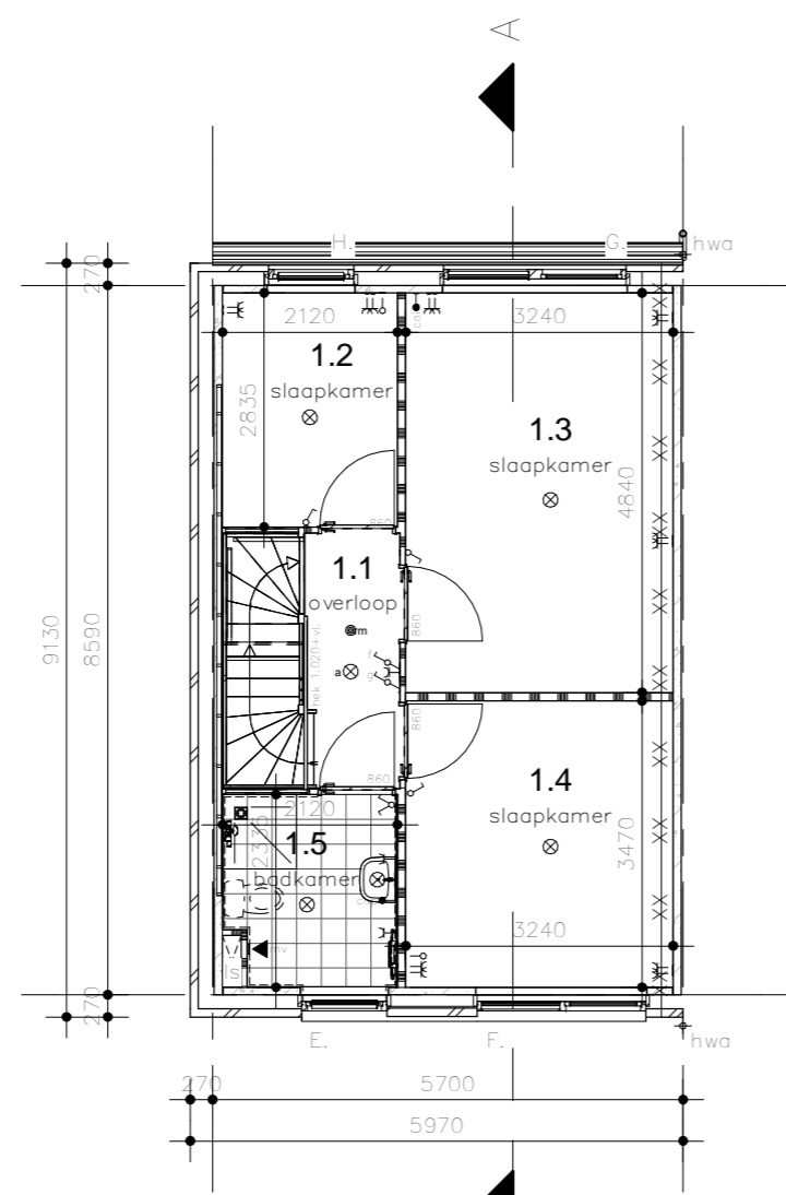
1e Verdieping (2.900+)
