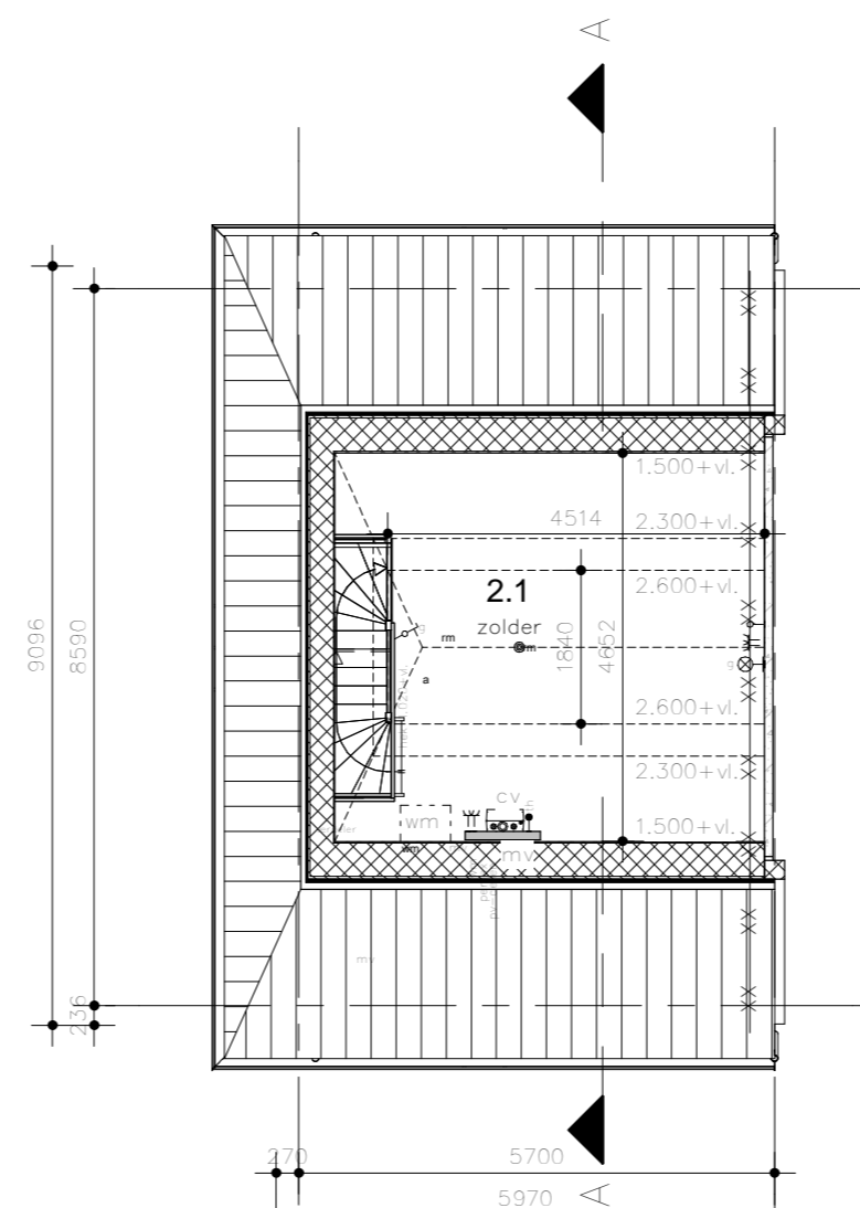
Zolder (5.800+)
