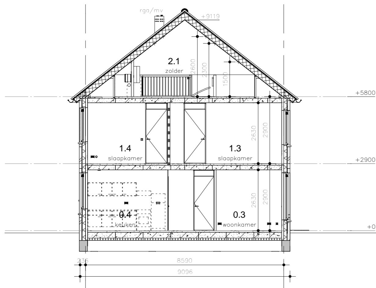
Doorsnede A-A
