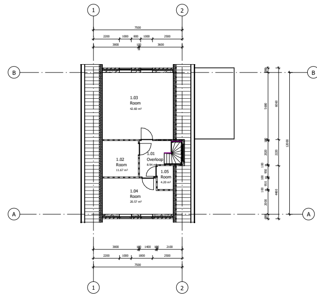
1e verdieping
