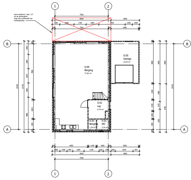
Begane grond
